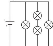
Kytentäkaavio C
