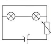
Kytentäkaavio E
