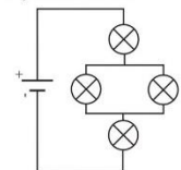
Kytentäkaavio D
